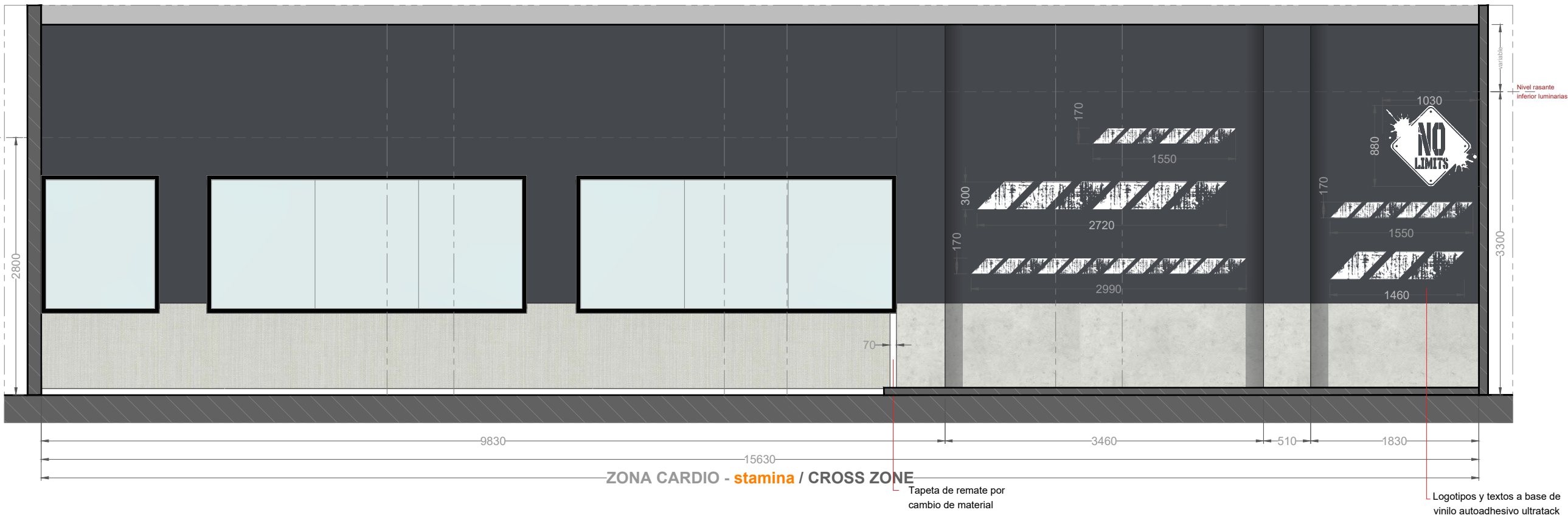
Alzado D | E: 1/50
