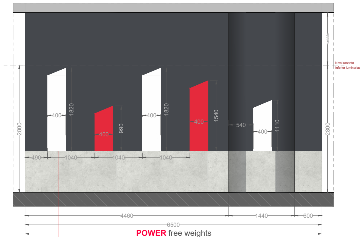
Alzado Z | E: 1/50
