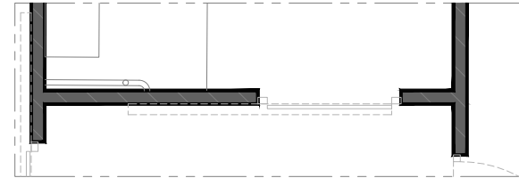
Alzado Z4 | E: 1/50
