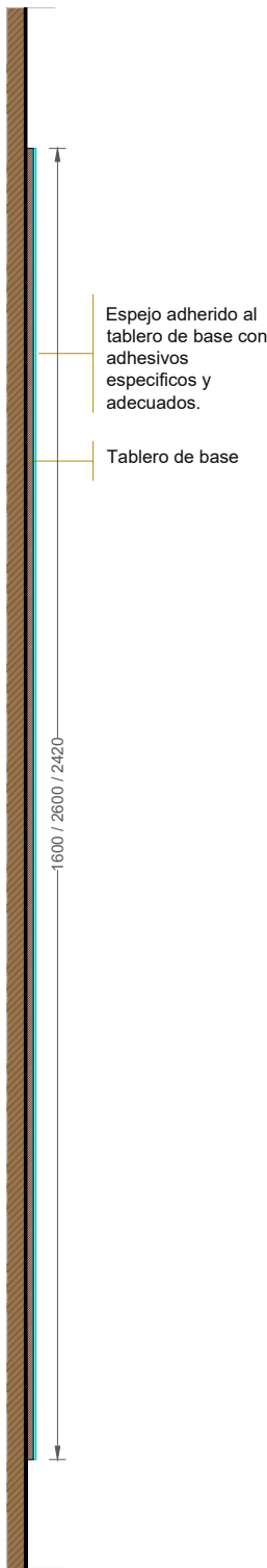
Sección espejos retranqueados | e: 1/15
