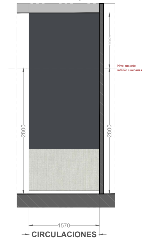
Alzado S | E: 1/50
