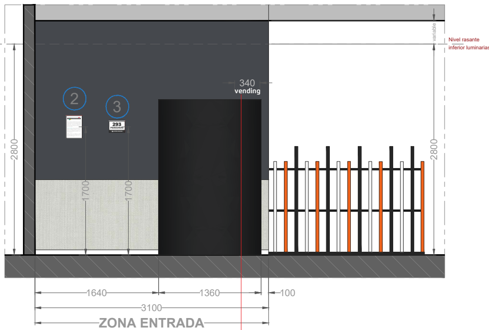
Alzado B | E: 1/50
