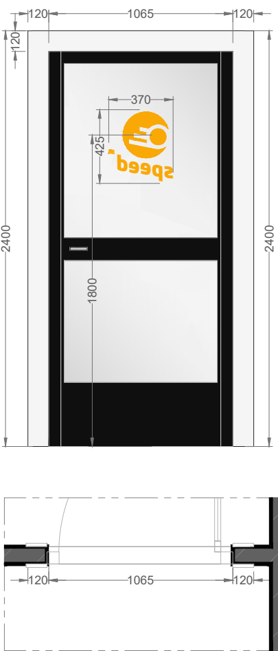
Detalle Pórtico | E: 1/10
