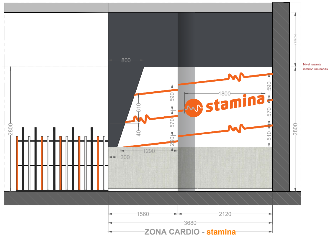
Alzado C | E: 1/50
