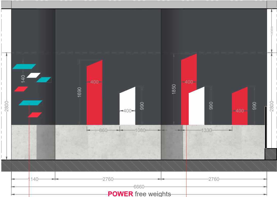
Alzado J | E: 1/50
