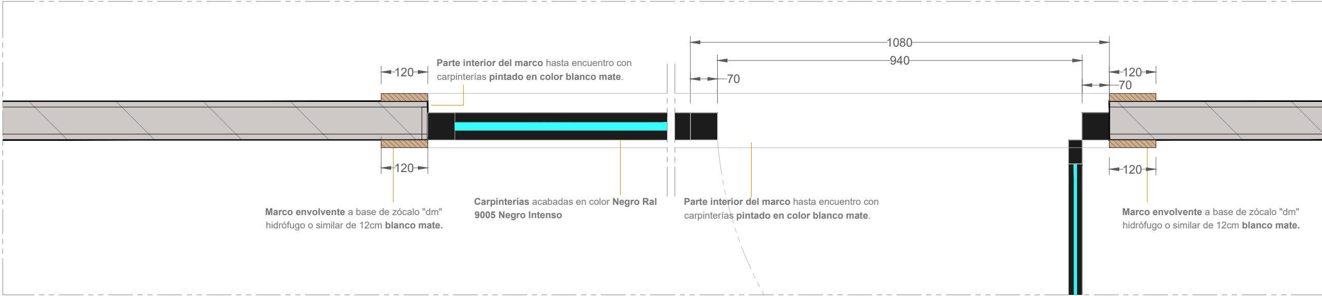
Detalle Pórtico | E: 1/10
