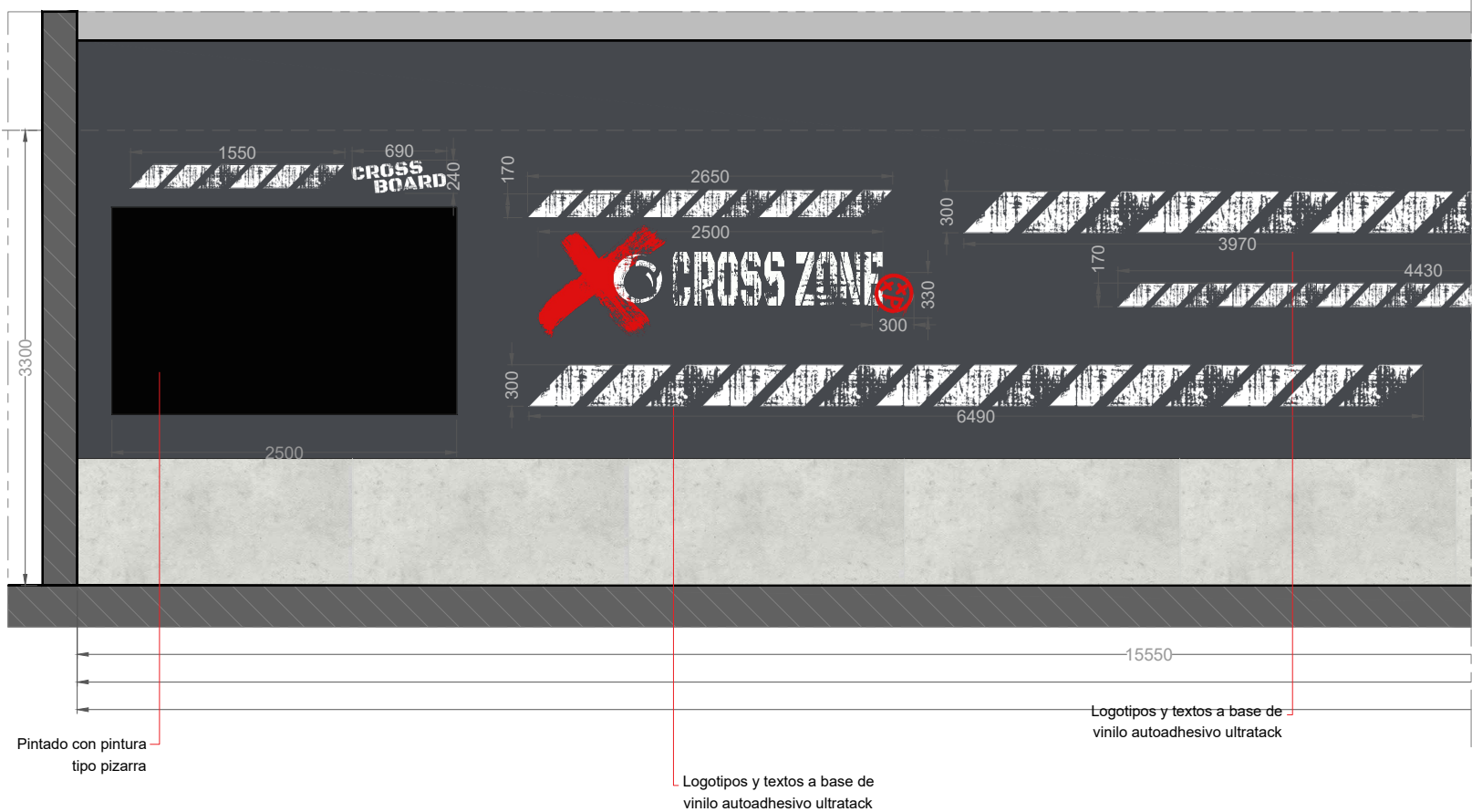
Alzado E | E: 1/50
